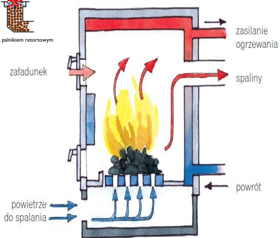
kocioł górnego spalania rozpalony od góry
