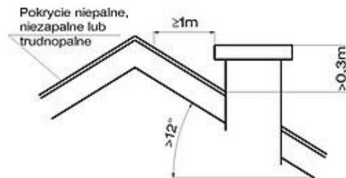
Rys.3. Przy dachach stromych o kącie nachylenia połaci dachowych powyżej 12° i pokryciu niepalnym, niezapalnym i trudno zapalnym, wyloty przewodów powinny znajdować się na wysokości co najmniej o 0,3 m wyżej od powierzchni dachu oraz w odległości mierzonej w kierunku poziomym od tej powierzchni co najmniej 1,0m.
