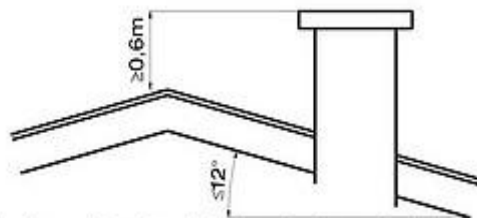
Rys.1. Przy dachach płaskich o kącie nachylenia połaci dachowych nie większym niż 12°, niezależnie od konstrukcji dachu, wyloty przewodów powinny znajdować się co najmniej o 0,6m wyżej od poziomu kalenicy lub obrzeży budynku przy dachach wgłębionych.
