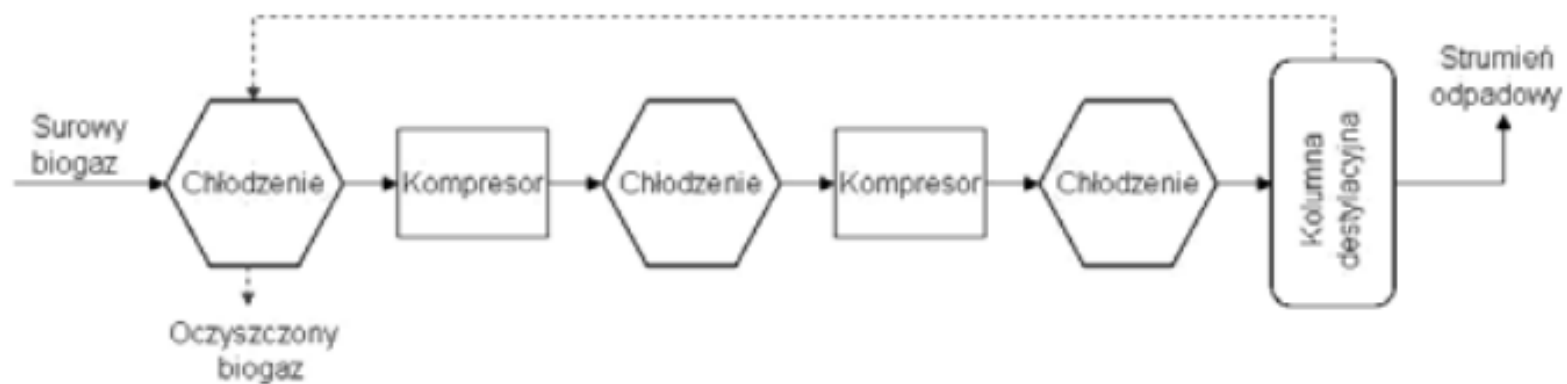
Schemat procesu separacji kriogenicznej
