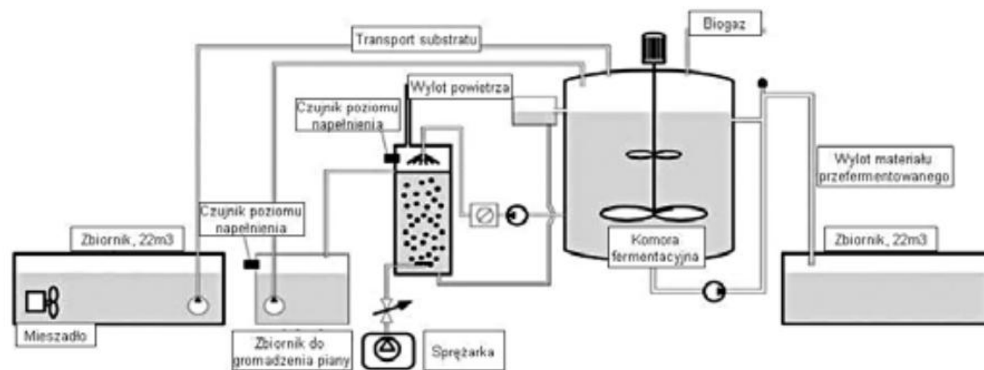
Schemat przebiegu wzbogacania metanu metodą in situ
