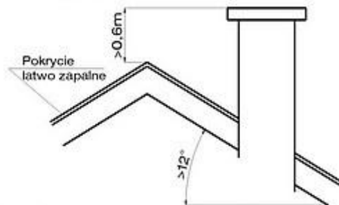
Rys.2. Przy dachach stromych o kącie nachylenia połaci dachowych powyżej 12° i pokryciu łatwo zapalnym, wyloty przewodów powinny znajdować się na wysokości co najmniej o 0,6m wyżej od poziomu kalenicy.
