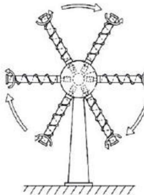
Rys.24. Siłownie wiatrowe wykorzystujące efekt Magnus'a: a) ACOWIND A-63, b) Mekaro Akita Co Ltd. (Japonia)
