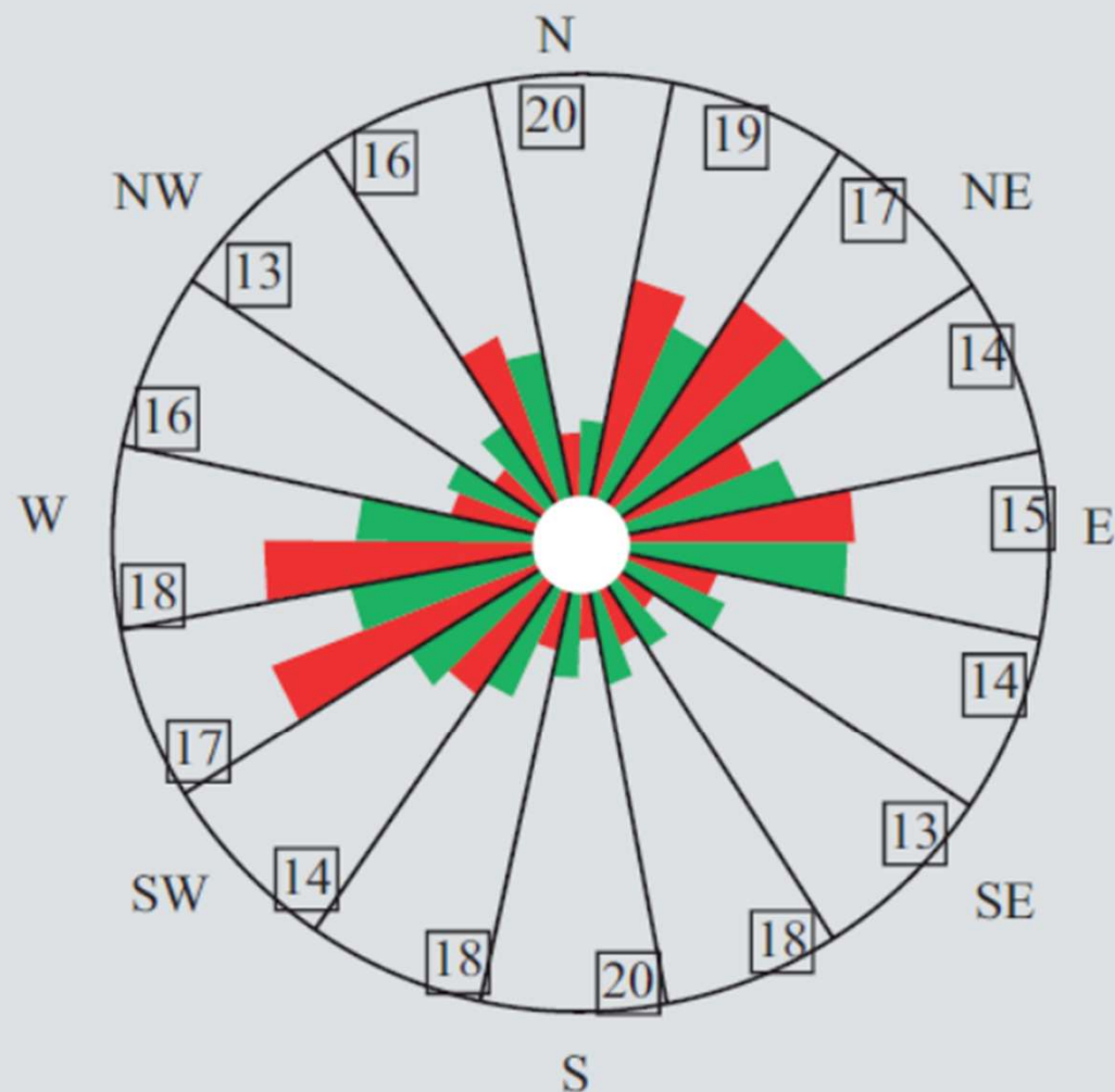
Róża wiatrów
