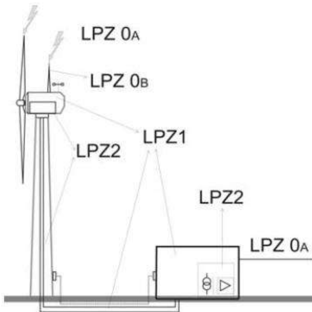
Rys. Rozmieszczenie stref ochronnych
