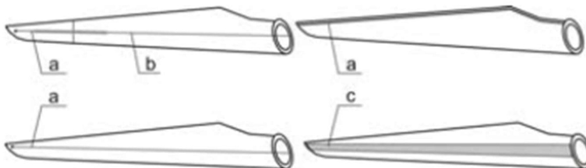
Rys. (po prawej) Stosowane rozwiązania dla przewodzenia prądu przez łopaty
