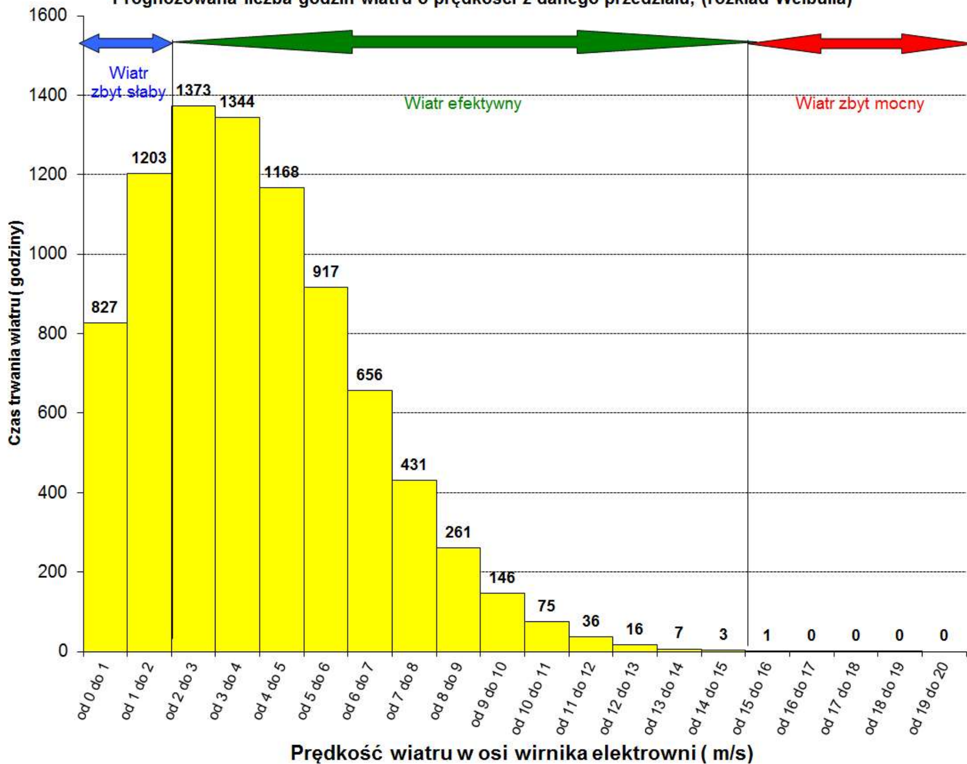
Prognozowana liczba godzin wiatru o prędkości z danego przedziału, (rozkład Weibulla)
