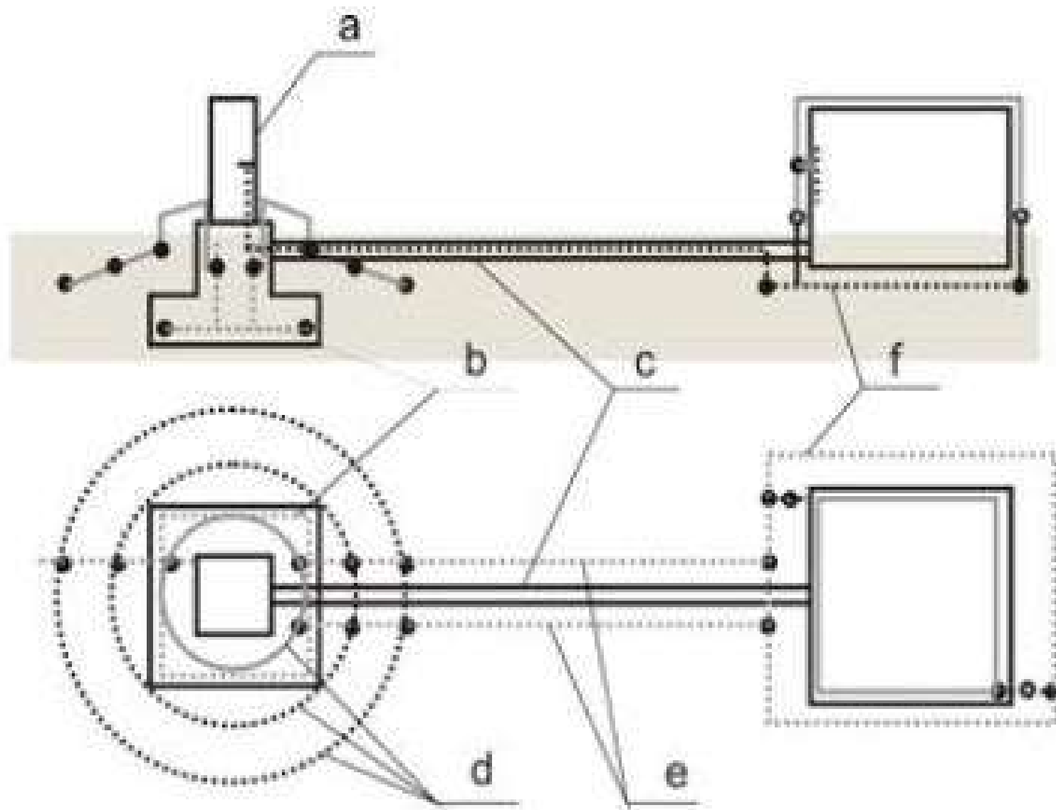
Rys. Rozmieszczenie uziomów elektrowni wiatrowej
