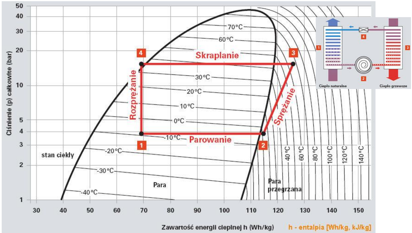
Rys. Diagram logarymiczny ciśnienie-entalpia dla R407C (pompa ciepła A/W)
