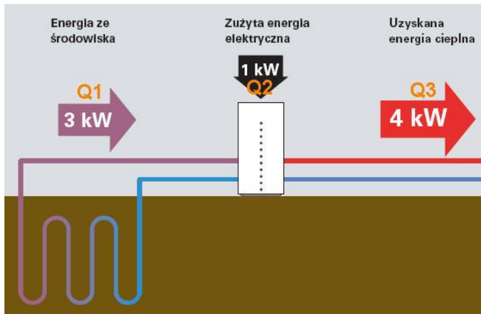
Rys. Przykładowy COP = 4 – ilość uzyskanej energii cieplnej jest 4 razy większa od zużytej energii elektrycznej; COP = 4 kW / 1 kW = 4
